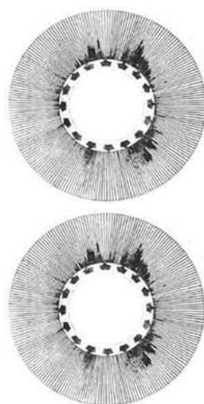
Рис. 24. План третьего яруса - купола храма. Реконструкция Т. Марутяна.
