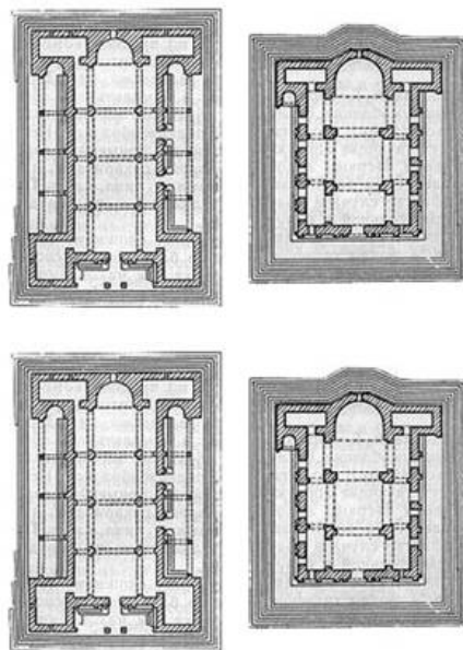
Рис. 1. Планы базилик в Еревуке и в Текоре (по Халпахчяну). (Воспроизведено по энцикл. «Всеобщая История Архитектуры», т. 3, 1970)
