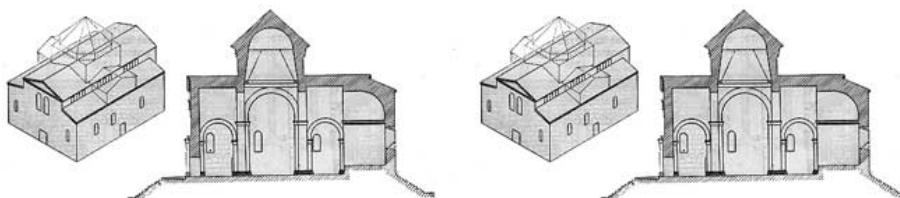
Рис. 3. Схематический разрез по оси север-юг и аксонометрия храма в Текоре (по Тораманяну). (Воспроизведено по энцикл. «Всеобщая История Архитектуры», т. 3, 1970)
