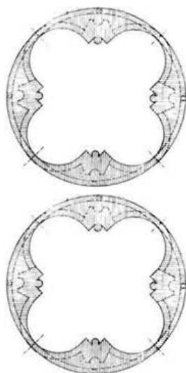
Рис. 26 Схема кольцевого каменно-бетонного блока. По Т. Марутяну.
