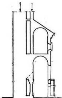
Рис. 27. Разрез по оси отдельно стоящей колонны позади пилона. По Т. Марутяну.
