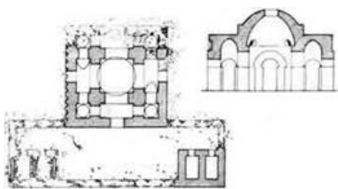
Рис. 12. Крестовокупольные храмы маздаистов IV - V вв. н.э. Чортак в Нейсаре. План и разрез. Храм Огня в долине Джерре. План, разрез. (Воспроизведено по энцикл. «Всеобщая История Архитектуры», т. 1, 1970)
