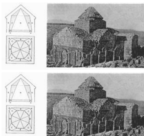
Рис. 4. План купола базилики в Текоре и общий вид до обрушения купола в 1912 г. (фото и план Тораманяна). Юго-западный фасад (воспроизведено по энцикл. «Всеобщая История Архитектуры», т. 3, 1970)
